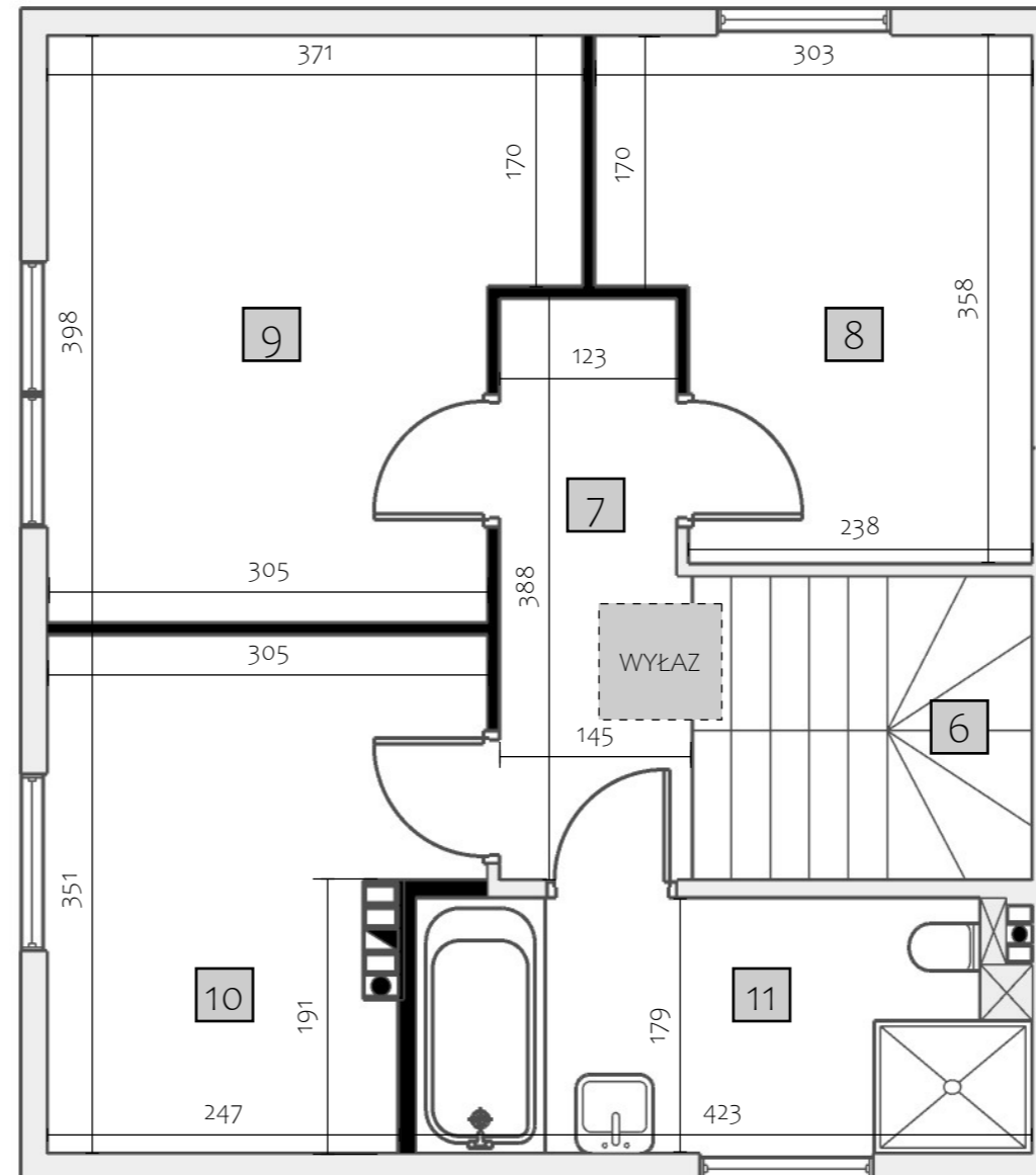
PIĘTRO H= 280
