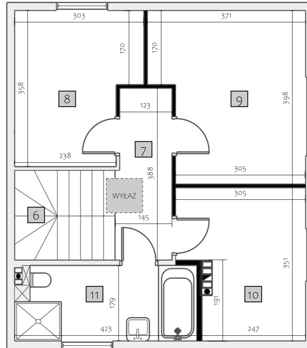
PIĘTRO H= 280
